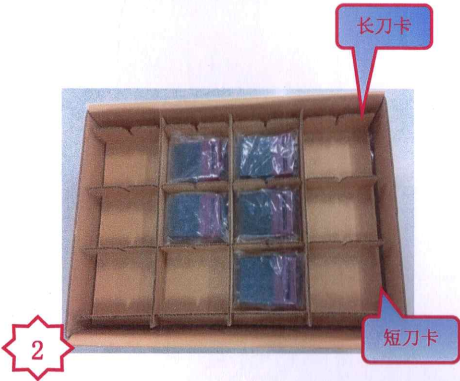
图二, 将 PA323 按照每层 12PCS, 每箱 3 层的方式进行包装, 同时在底层和每层的顶部放一块隔板, 共 4 块隔板。
